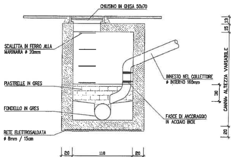
SEZIONE A-A
