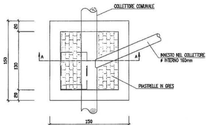
PIANTA
