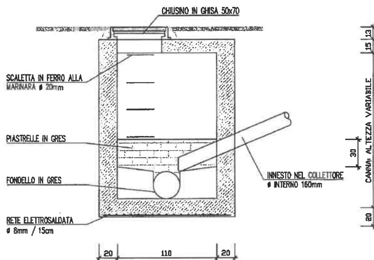
SEZIONE A-A
